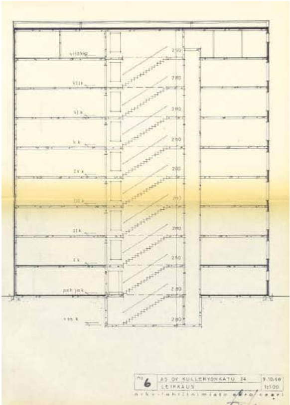
LEIKKAUS
