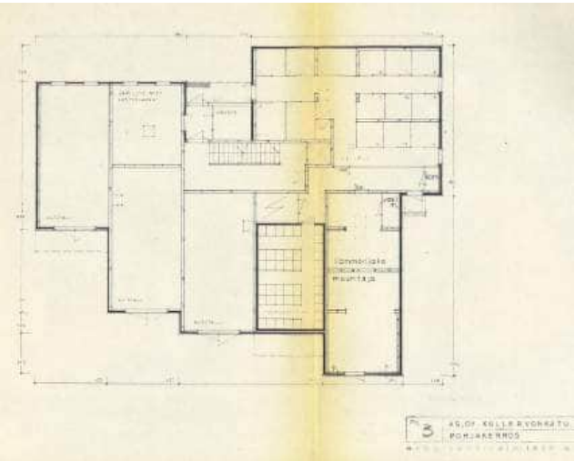
P-Krs. Katutaso
