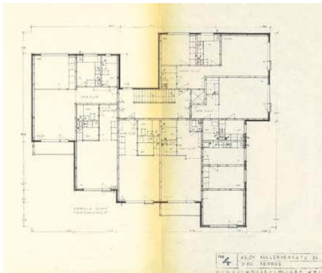
Asuinkerrokset 1-7
