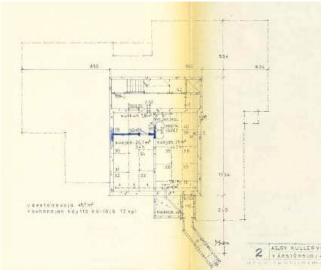
KELLARI
