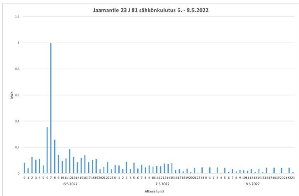
Kaavio 1: Jaamantie 23 J 81 sähkönkulutus 6. - 8.5.2022
