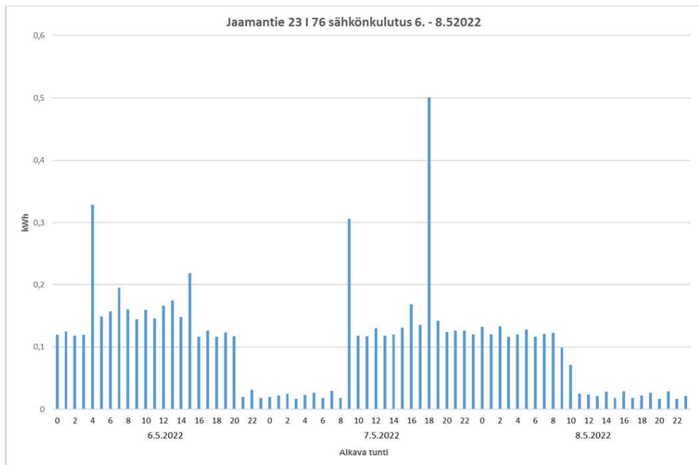
Kaavio 2: Jaamantie 23 I 76 sähkönkulutus 6. - 8.5.2022
