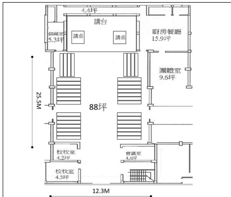
平面圖
