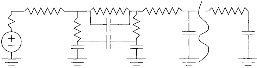
Figure 4.11. A simple RC-circuit.
