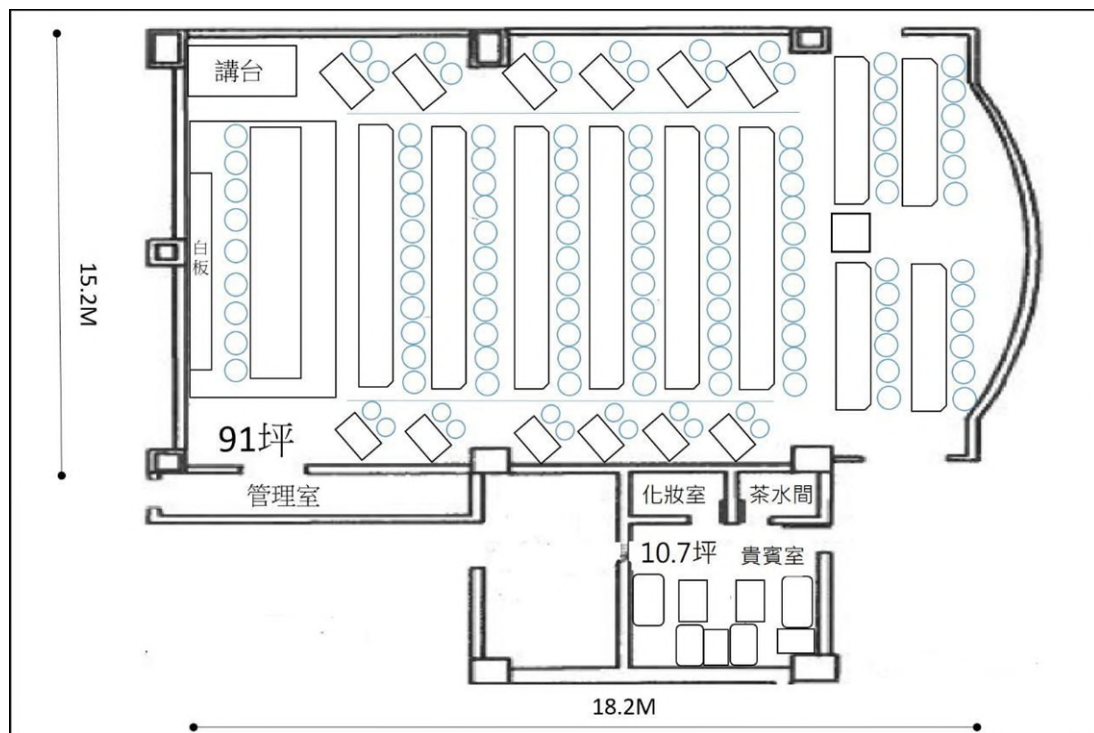
平面圖
