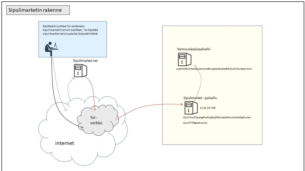
Kuva Sipulimarket -sivuston teknisestä rakenteesta
